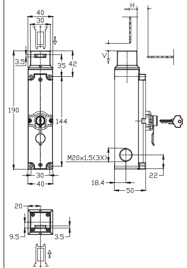
Dimensioni (mm)
