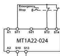
Fig. 5: Arresto di emergenza a due canali circuito con cortocircuito con monitoraggio dei guasti a terra (fino alla categoria 3, PL d, SIL 2)
