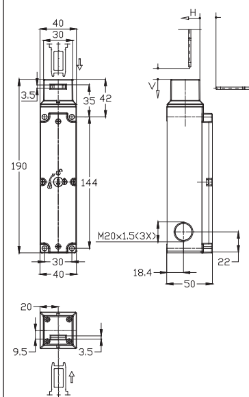
Dimensioni (mm)
