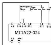
Fig. 4: Arresto di emergenza a due canali circuito con cortocircuito con monitoraggio dei guasti a terra (fino alla categoria 4, PL e, SIL 3)
